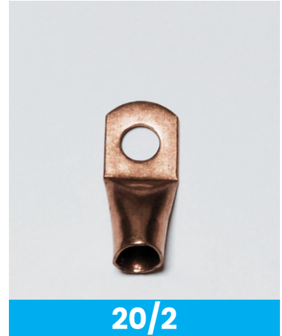
20/2 Terminal para cable de 35 mm aguj. de 10mm
